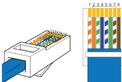
Zapojenie CAT kábla do RJ45
